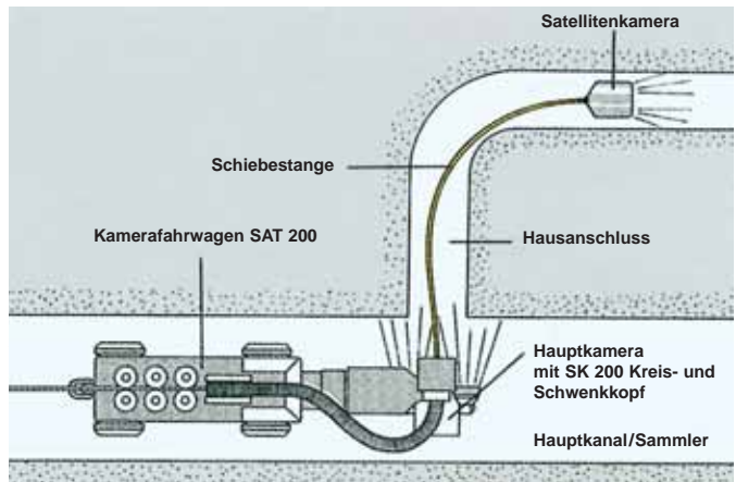
Satellitenkameranystem
